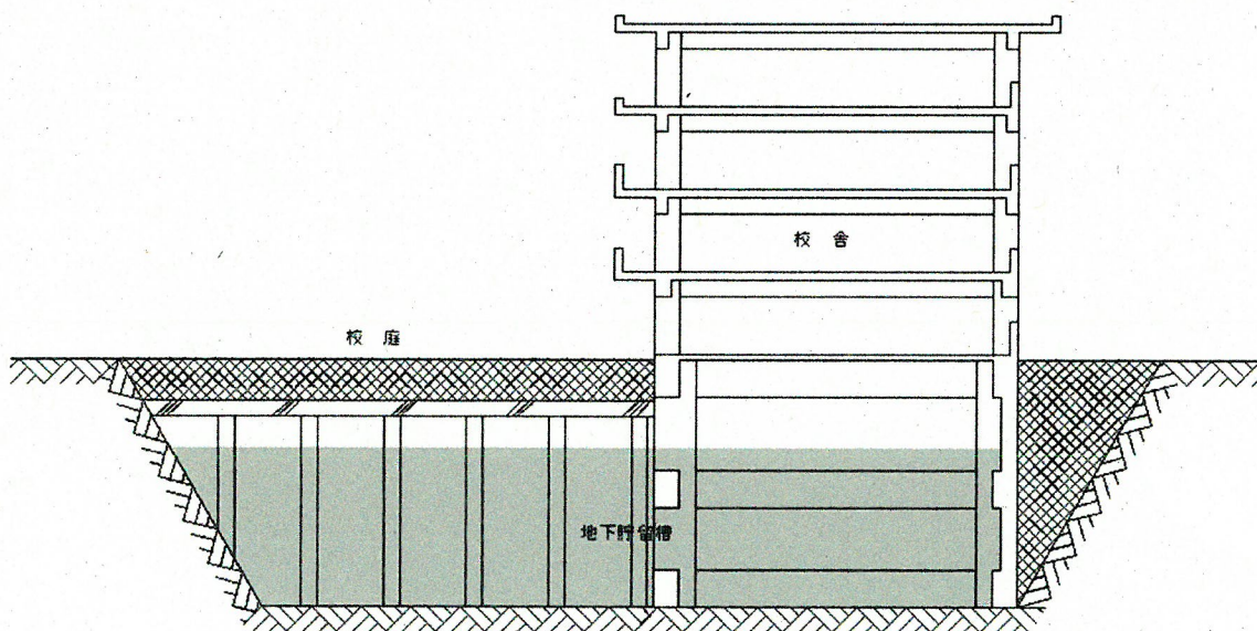
本地区調整池における地下貯留槽のイメージ断面図
